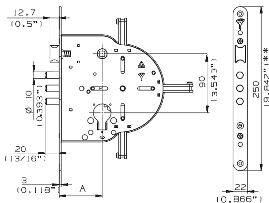
Модель 235 многоканального замка с 6 засовами
