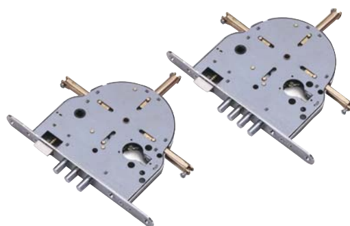
Модель 235 многоканального замка с 6 засовами
