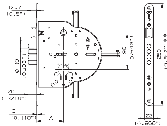
Модель 265 многоканального замка с 7 засовами
